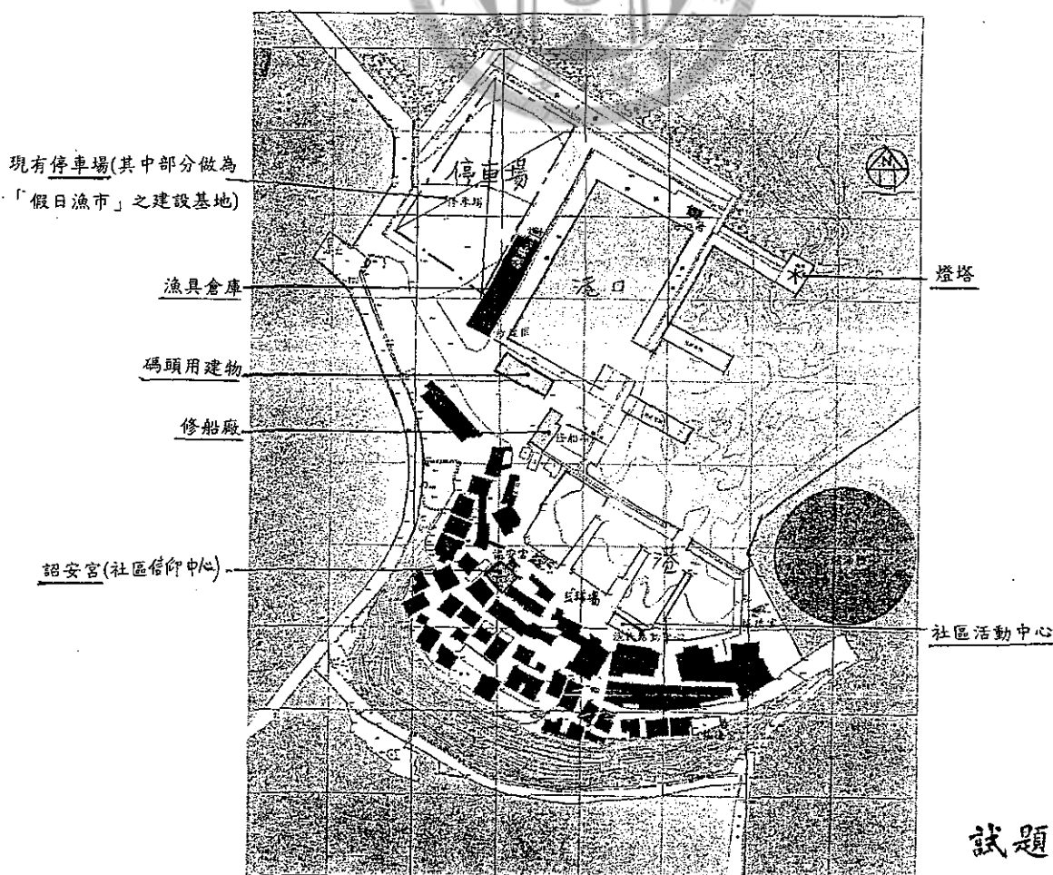
漁港及漁村全區配置圖
